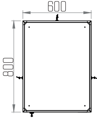
ÜST GÖRÜNÜŞ
