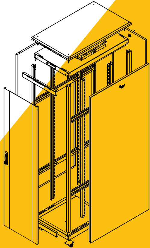
İZOMETRİK PATLATILMIŞ GÖRÜNÜŞ
